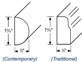
Countertop Edge
